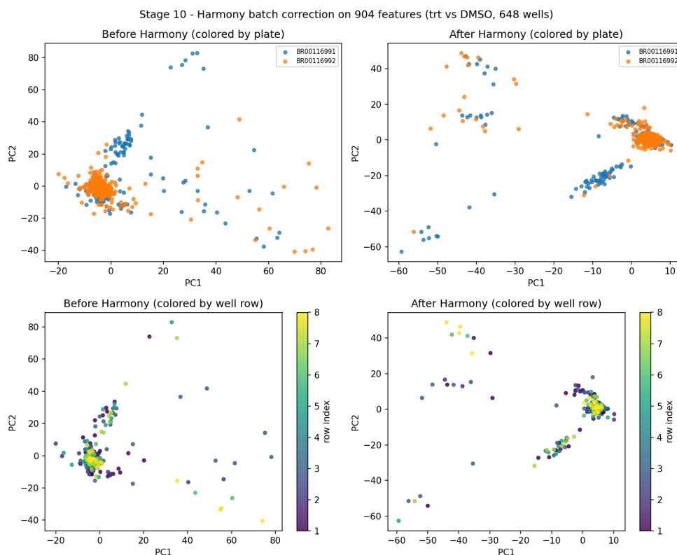
Harmony batch correction PCA
