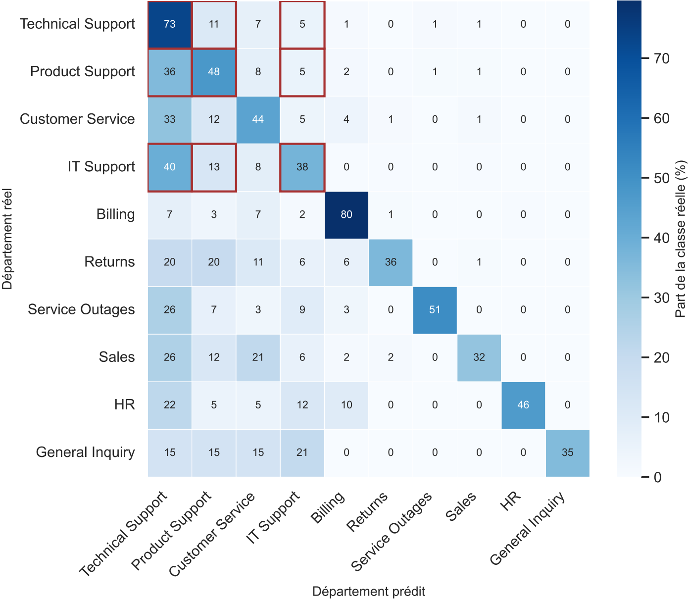
Matrice de confusion du modèle de département
