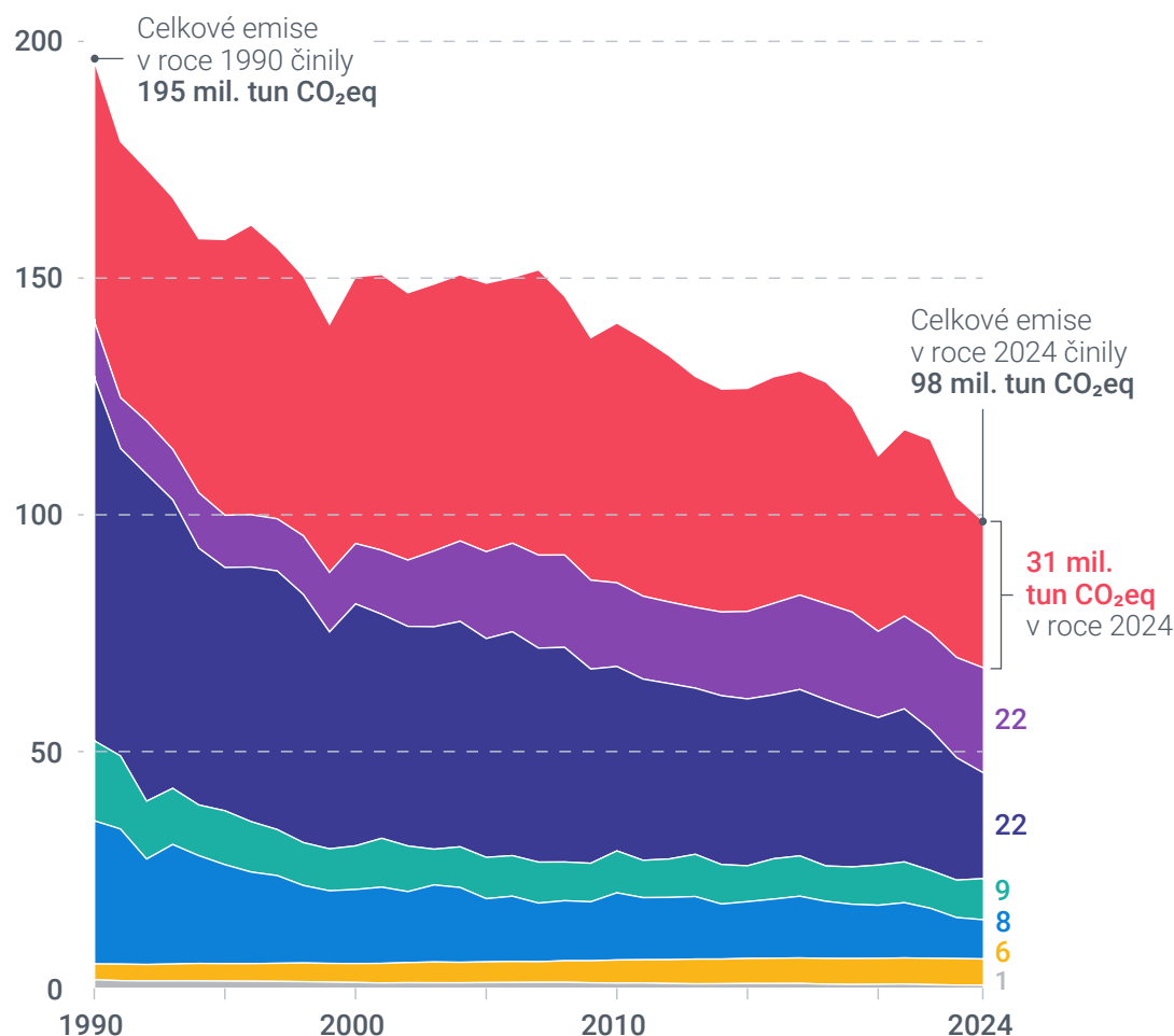
VÝVOJ EMISÍ v letech 1990–2024
