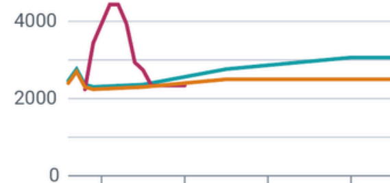
Benzín Kč/l
