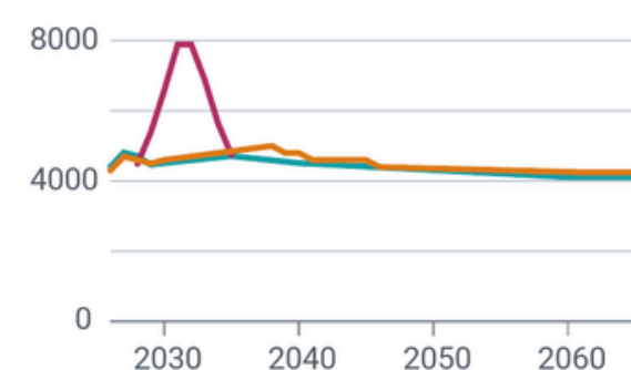
Elektřina Kč/MWh
