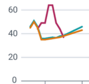
Benzín Kč/l
