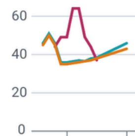
Nafta Kč/l
