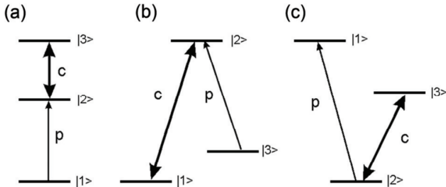
Rysunek: Najprostsze konfiguracje EIT: a) kaskadowa (drabinowa), b) \Lambda , c) V. Oznaczono: p – laser próbkujący, c – silne sprzężenie (za: Kowalski et al., 2010)
