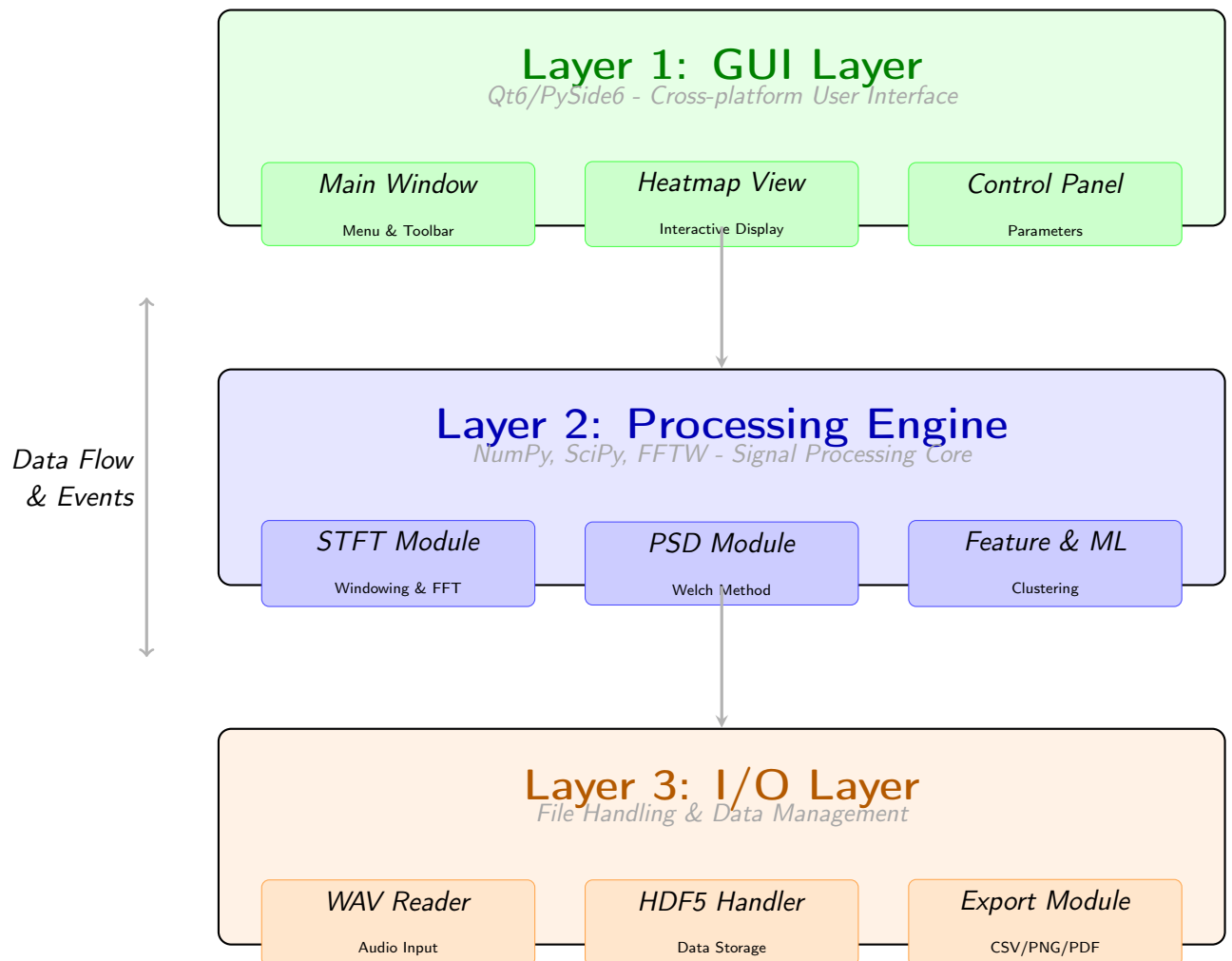
Gambar 22: Arsitektur 3-Layer Sistem Pertacoustic
