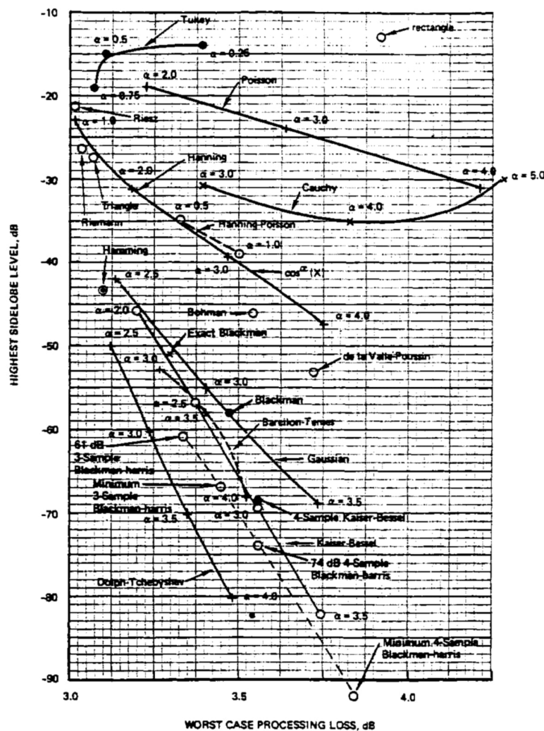
Gambar 20: Perbandingan karakteristik berbagai window functions menurut [10]. Grafik menunjukkan trade-off antara main lobe width (resolusi frekuensi) dan side lobe level (spectral leakage). Hann window dipilih untuk sistem Pertacoustic karena memberikan balance optimal. Sumber: Proceedings of the IEEE , 66(1), 51-83.
