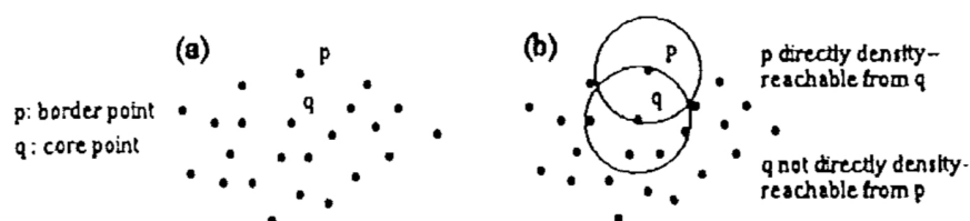
Gambar 21: Ilustrasi DBSCAN algorithm menurut [17]. (a) Menunjukkan core points dan border points dalam clustering. (b) Menunjukkan konsep density-reachability. Algoritma ini dapat menemukan clusters dengan bentuk arbitrary dan mengidentifikasi outliers sebagai noise, fitur kritis untuk anomaly detection seperti channeling dan leaks dalam sistem SNL. Sumber: Proceedings KDD-96 , 226-231.
