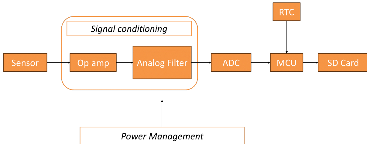
Gambar 2: Desain skema data logger
