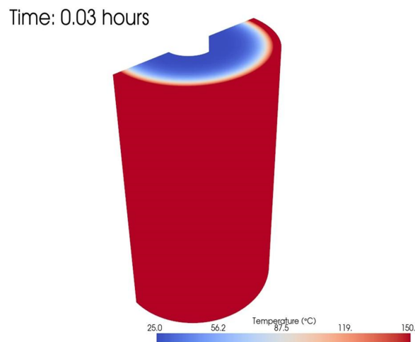
Gambar 18: Animasi 3D hasil akhir pemodelan
