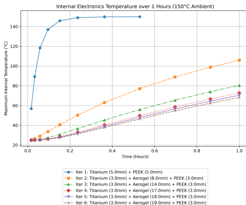
Gambar 17: Hasil analisis termal dengan beberapa kombinasi bahan
