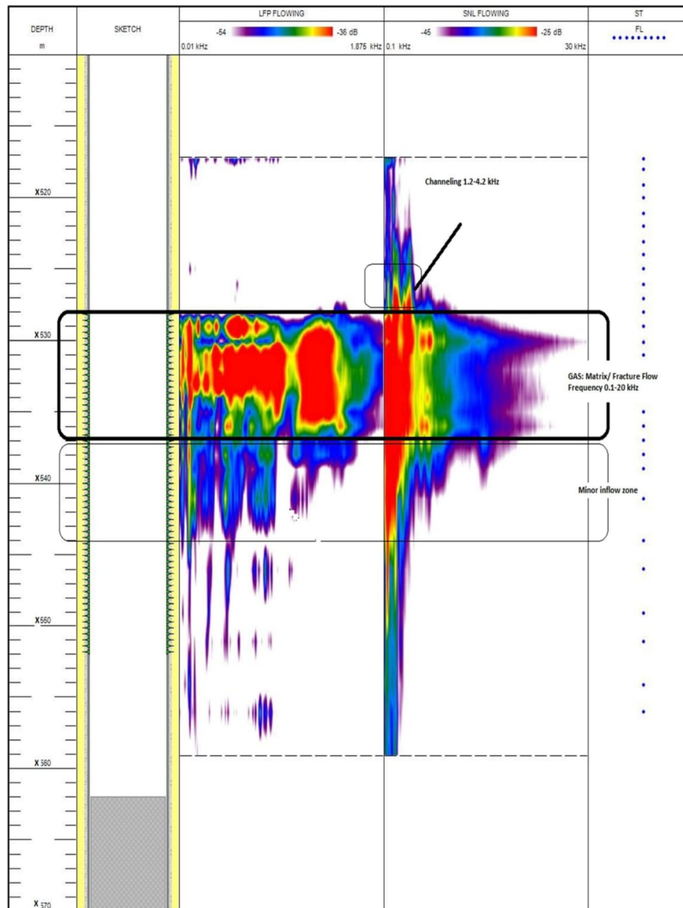
Gambar 19: Depth-frequency heatmap dari [3] yang menunjukkan metodologi visualisasi untuk sistem Pertacoustic. Sumbu vertikal merepresentasikan depth, horizontal merepresentasikan frequency, dan intensitas warna merepresentasikan amplitude sinyal akustik. Format ini terbukti sangat efektif untuk interpretasi oleh engineer lapangan. Sumber: Journal of Petroleum Science and Engineering , 206, 109005.
