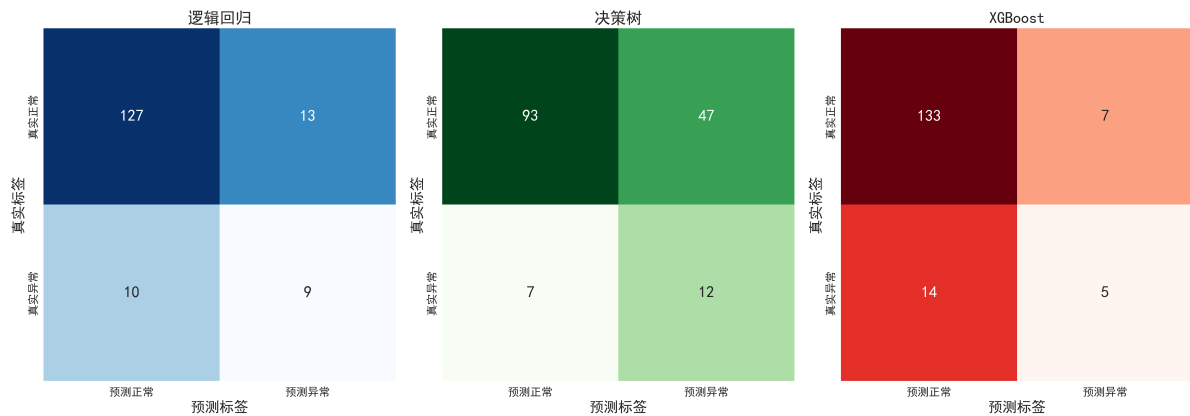
图 30 模型混淆矩阵对比
