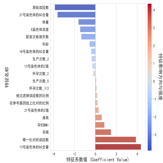
图 31 逻辑回归模型特征系数排序
