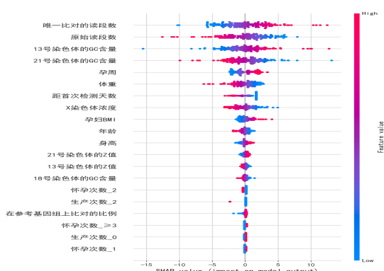
图 32 SHAP 摘要图
