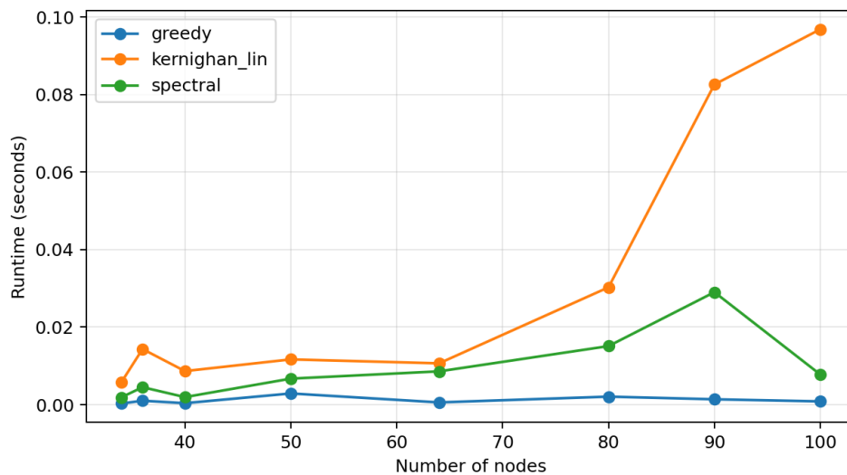
图 2: 运行时间对比。贪心最快；Kernighan-Lin 需要额外细化时间。
