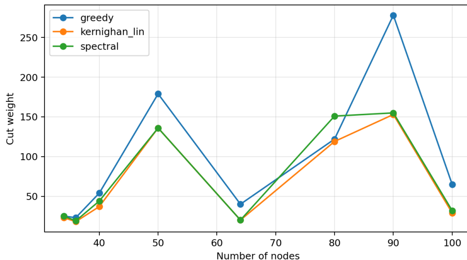
图 1: 割边权重对比。数值越低，表示跨工作节点通信越少。
