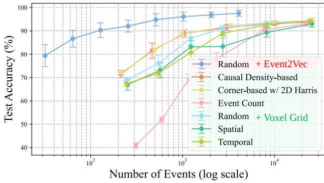
Figure 3. 在 DVS Gesture 数据集上，与 (Araghi et al., 2025) 中采样技术相比的精度-事件数量关系。
