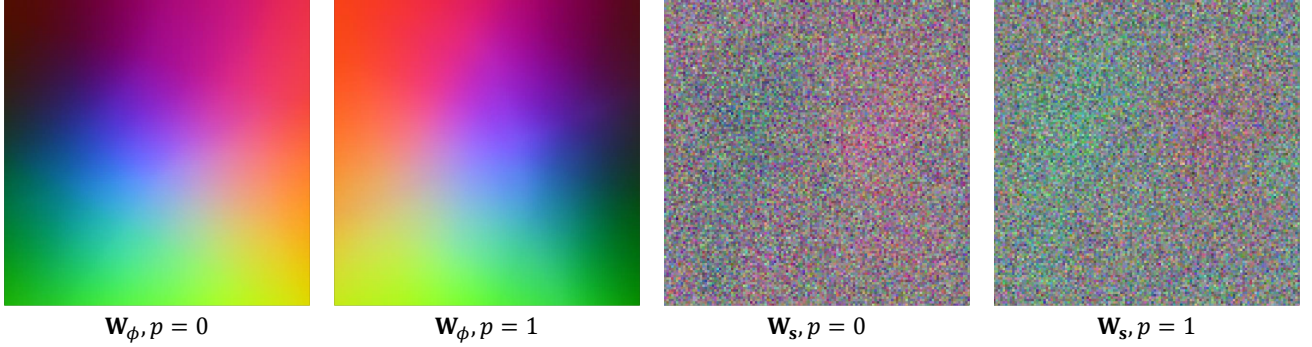
Figure 8. RGB 域中参数化嵌入权重 \mathbf{W}_\phi 与标准嵌入权重 \mathbf{W}_s 的可视化。
