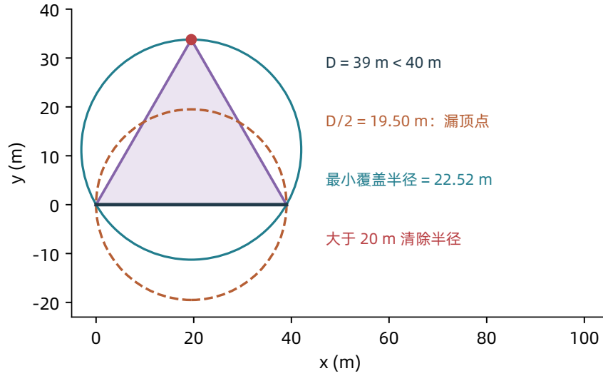
图 3: 直径小于 40 m 仍不能由一个 20 m 清除圆覆盖。紫色为等边三角形定位区域，橙色虚线圆以最长边为直径，蓝色实线圆是最小覆盖圆。关键是最小所需半径 22.52 m 仍超过清除半径，不能仅检查区域直径。
