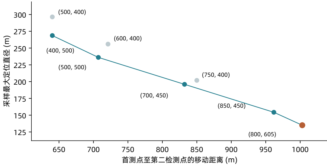
图 6: 定位精度与移动距离的权衡。展示固定库的全部 8 个上侧候选, 镜像具有相同指标; 蓝色为库内非支配点, 灰色为被支配候选, 橙色突出 (800,605)。纵轴是有限场景的最大值, 不是置信上界。
