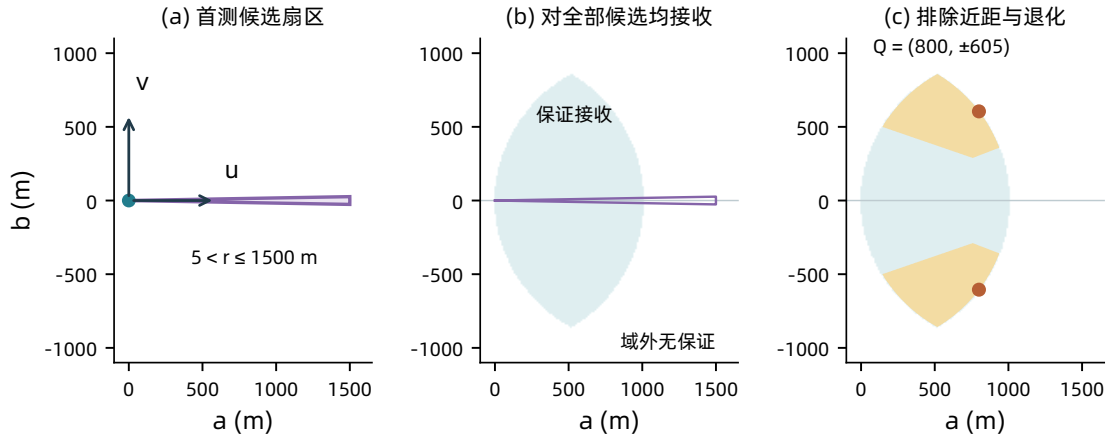
图 5: 第二测点选择的三个步骤。(a) 紫色窄扇区表示首次测向候选源；(b) 浅蓝色表示对整个外包扇形保证接收，域外仅表示没有该保证，紫线附近还需排除潜在 5 m 近距情形；(c) 浅黄色进一步满足式 (8)，橙点为选定镜像候选。三图同尺度，显示网格不承担证明。
