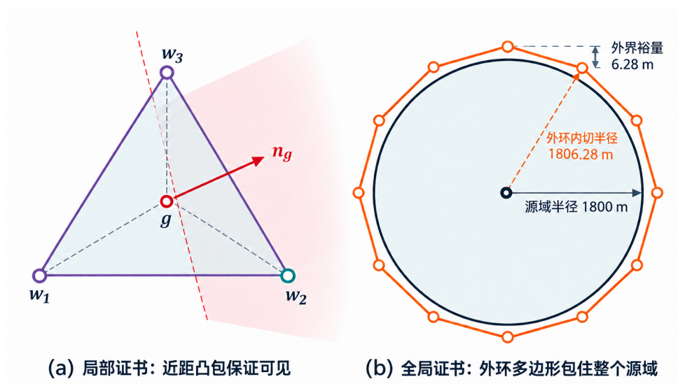
图 13: 定向源发现保证的局部与全局几何示意。(a) 源位于近距站的凸包内，任意发射方向至少有一个站可见；(b) 外环正十二边形包围半径 1800 m 的源域，内切半径为 1806.28 m。图不按比例绘制；内切半径指圆心到边的垂距，顶点到圆心的外环半径为 1870 m。
