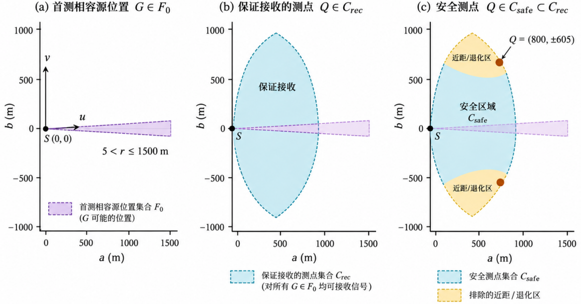
图 5: 第二测点候选区域的构造示意。(a) 首次测向的相容源位置; (b) 保证接收的测点集合; (c) 安全测点筛选及推荐镜像点。填色仅示意集合关系, 不作为边界或点归属的数值判断; 安全区域严格由式 (7) 和式 (8) 共同确定, 轴线上退化测点不属于安全区域。
