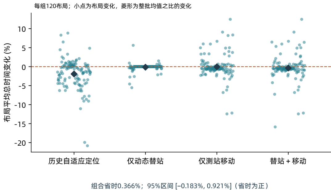
图 20: Q4 最新锁定验证的布局配对分布。每组 120 个点，每点合并同一布局 8 种误差与舍入条件；纵轴为时间变化，正值表示变慢。深色菱形是整批均值之比的变化，不是各点的简单平均；下方区间以“省时为正”报告组合的主要效应。
