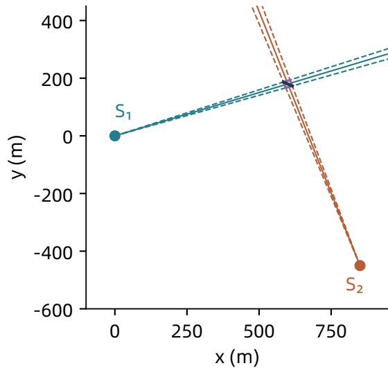
(a) 两条 \pm 1^\circ 测向扇区
