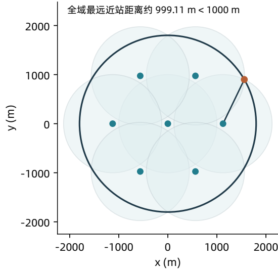
图 10: 七站对全向源的连续发现覆盖。浅蓝圆盘为各站 1000 m 的保证接收范围, 黑色圆为源域边界; 边界标点示意最不利角位置。覆盖依据为式 (11), 并非图上圆盘看似相接。
