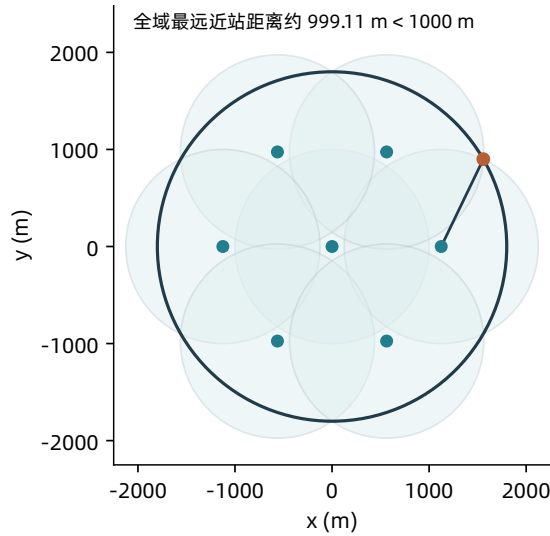
图 10: 七站对全向源的连续发现覆盖。浅蓝圆盘为各站 1000 m 的保证接收范围，黑色圆为源域边界。式 (11) 对整个连续圆域成立；穿插源服务任务时仍保留各频道的实际扫描记录。
