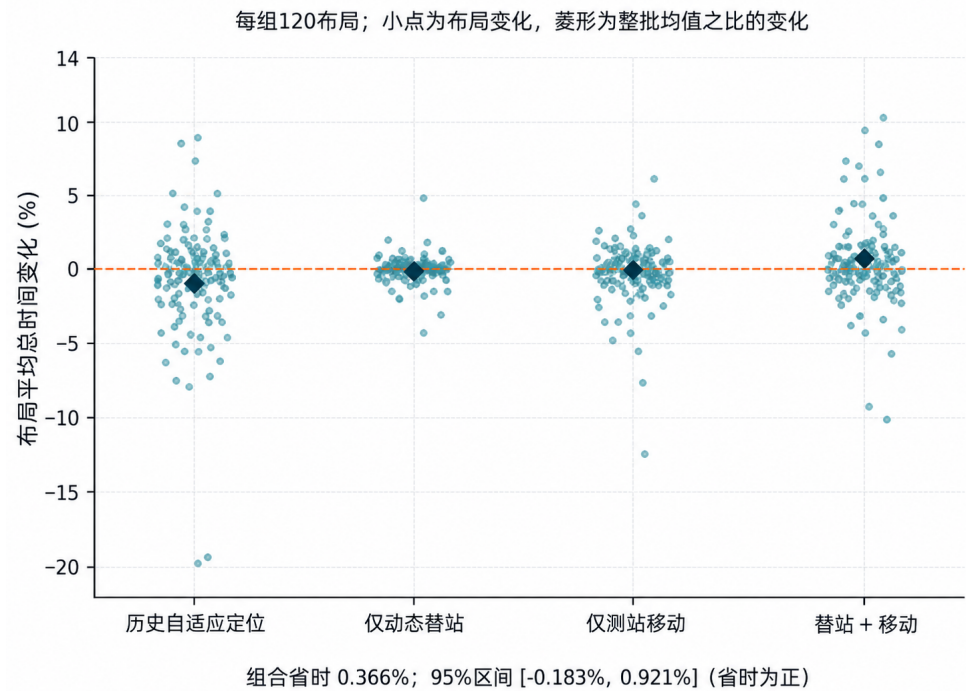
图 20: Q4 最新锁定验证的布局配对分布示意。每组对应 120 个布局，每个布局合并 8 种误差与舍入条件；纵轴为总时间变化，正值表示变慢，下方以省时为正报告效应区间。图中部分点位与核验统计存在偏差，组合菱形对应时间变化 -0.366%，而非正值；精确配对结果以正文及源数据为准。
