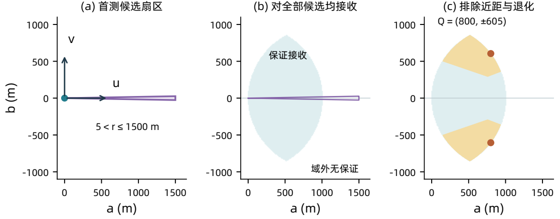
图 5: 第二测点选择的三个步骤。(a) 紫色窄扇区表示首次测向候选源；(b) 浅蓝色表示对整个外包扇形保证接收，域外仅表示没有该保证，紫线附近还需排除潜在 5 m 近距情形；(c) 浅黄色进一步满足式 (8)，橙点为选定镜像候选。三图同尺度，显示网格不承担证明。
