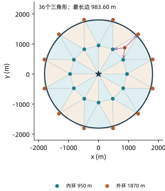
图 12: 25 站双环搜索构造。中心站与内、外环分别位于 0、950 和 1870 m 处, 两环错开 15°, 连接形成 36 个三角形。最长边小于 1000 m, 外环正多边形包围目标圆域, 从而对任意源位置和发射方向提供发现保证。
