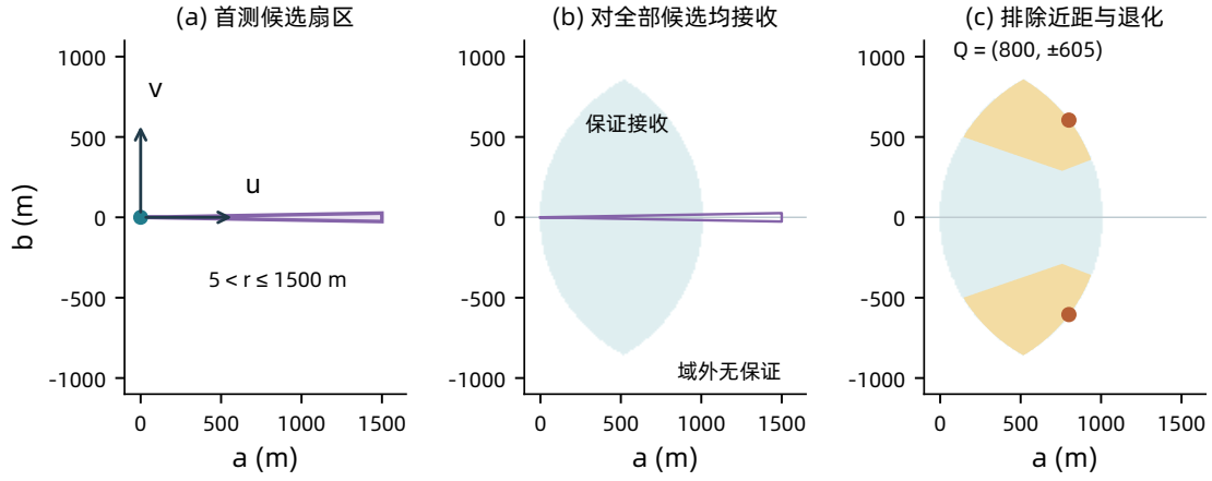
图 5: 第二测点候选区域的构造。(a) 首次测向的完整候选扇形; (b) 满足式 (7) 的保证接收区域; (c) 进一步满足式 (8) 的安全区域及优选镜像点。填色网格用于显示, 连续保证来自解析不等式。
