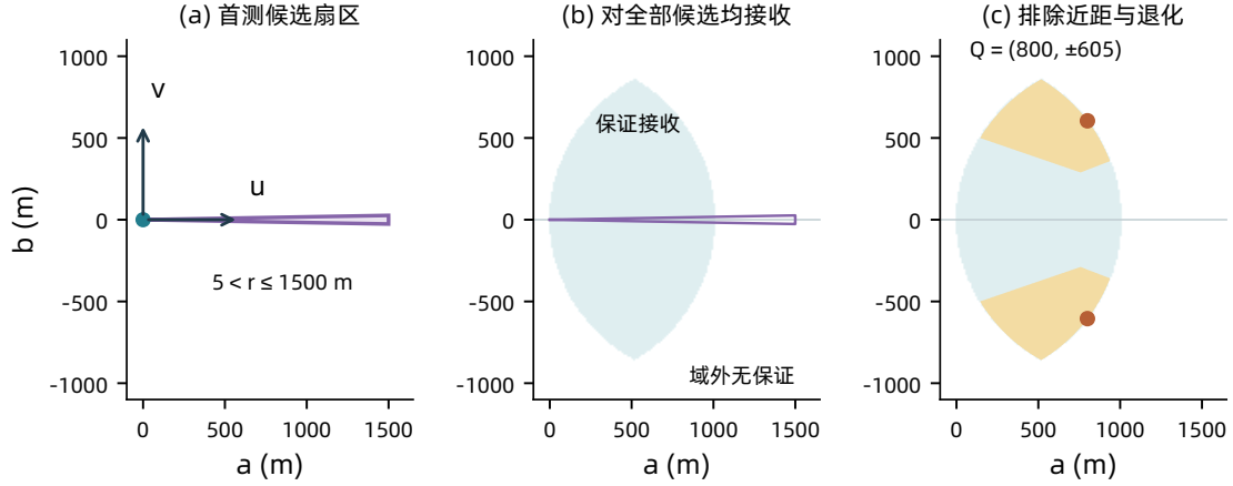
图 5: 第二测点选择的三个步骤。(a) 紫色窄扇区表示首次测向候选源；(b) 浅蓝色表示对整个外包扇形保证接收，域外仅表示没有该保证，紫线附近还需排除潜在 5 m 近距离情形；(c) 浅黄色进一步满足式 (8)，橙点为选定镜像候选。三图同尺度，显示网格不承担证明。
