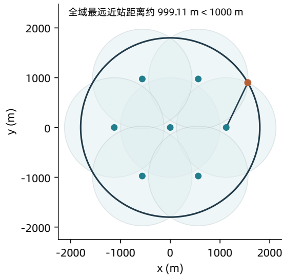
图 10: 七站对全向源的连续发现覆盖。浅蓝圆盘为各站 1000 m 的保证接收范围，黑色圆为源域边界。式 (11) 对整个连续圆域成立；穿插源服务任务时仍保留各频道的实际扫描记录。
