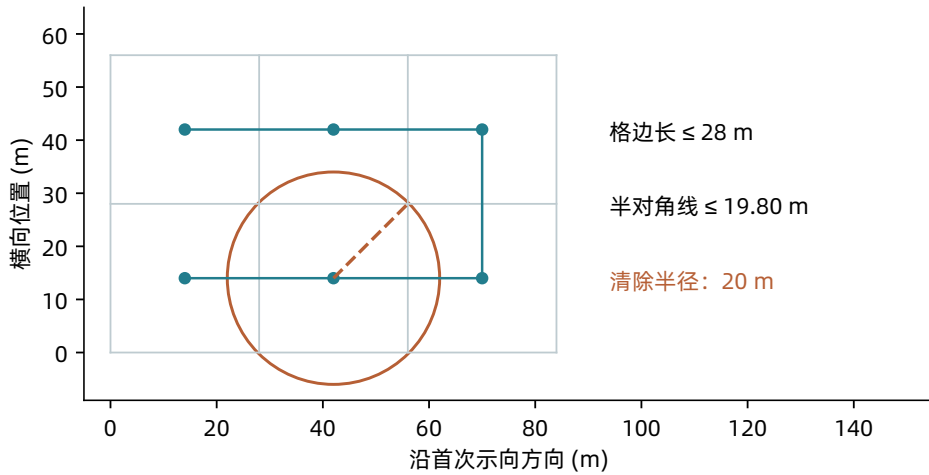
图 13: 有限光学网格。每格两边不超过 28 m，因此格心的 20 m 清除圆覆盖整个格。图示六格局部区域及蛇形访问顺序，实际格数由当前位置区域决定，清除成功后停止访问。
