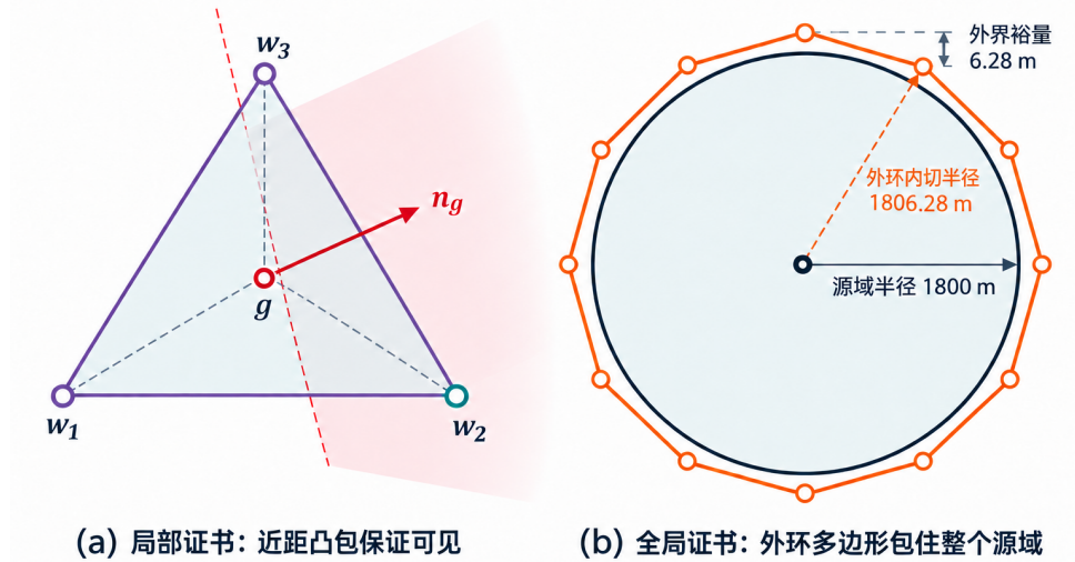
图 13: 定向源发现保证的局部与全局几何示意。(a) 源位于近距站的凸包内，任意发射方向至少有一个站可见；(b) 外环正十二边形包围半径 1800 m 的源域，内切半径为 1806.28 m。图不按比例绘制；内切半径指圆心到边的垂距，顶点到圆心的外环半径为 1870 m。
