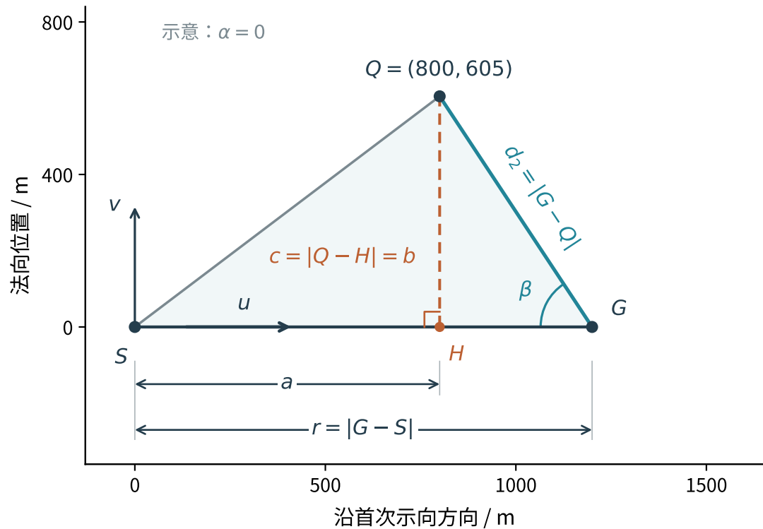
(a) 交会三角形与横向距离
