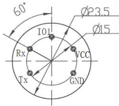
图 4 模组仰视尺寸图
