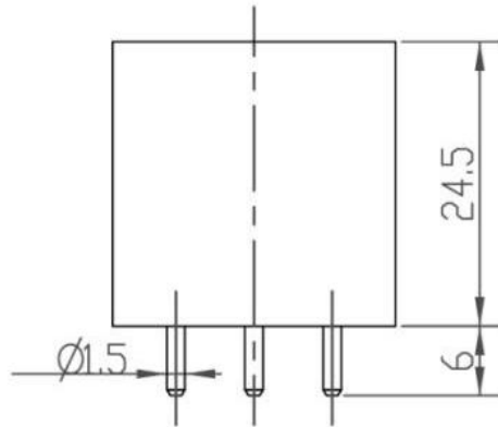
图 3 模组外观尺寸图
