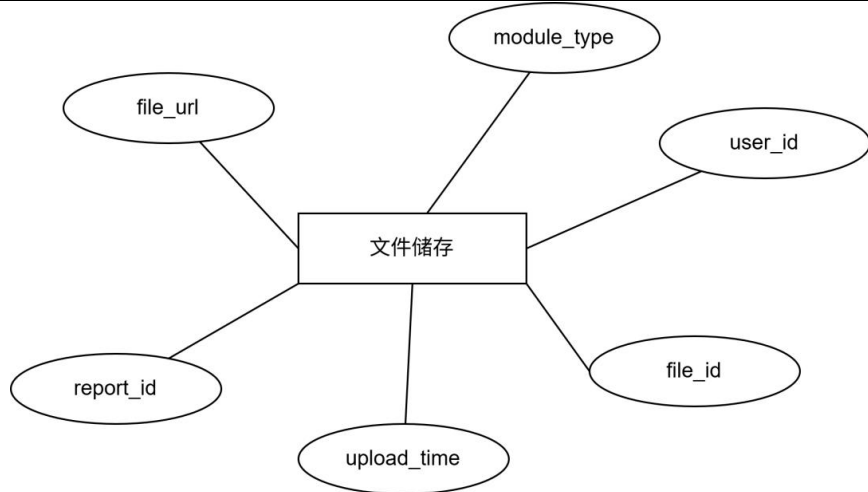
图 3-7 文件储存数据库设计
