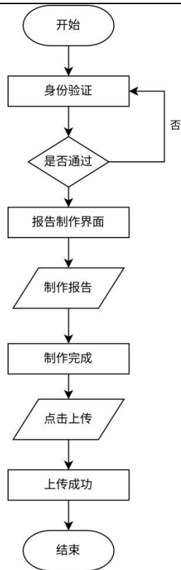
图 3-14 上传报告流程图
