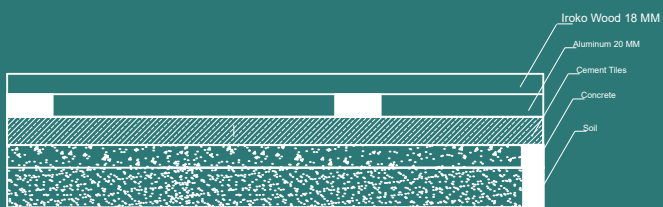
SEC D-D
