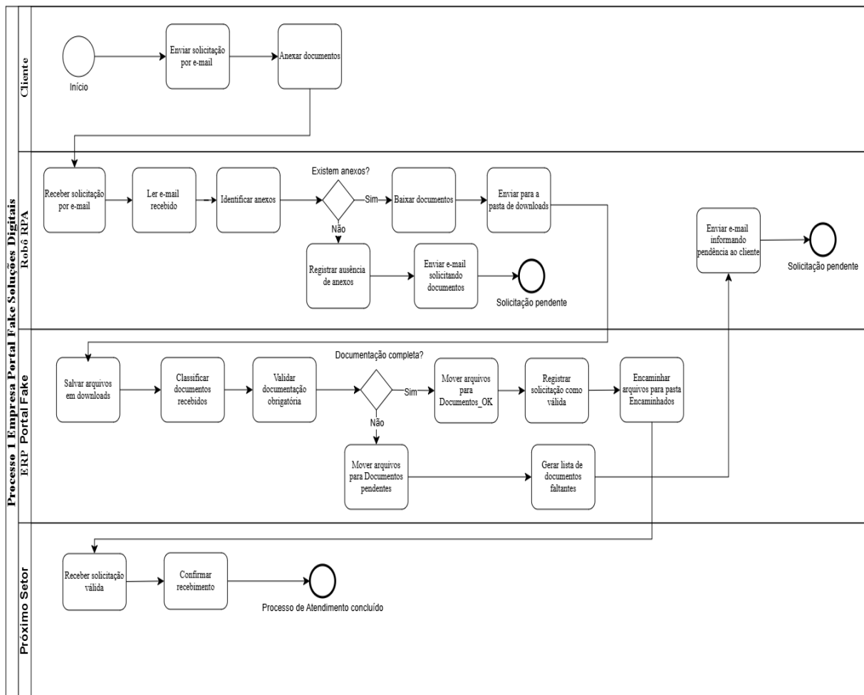
Figura 1 – BPMN do Processo 1: Atendimento da Empresa Portal Fake.
