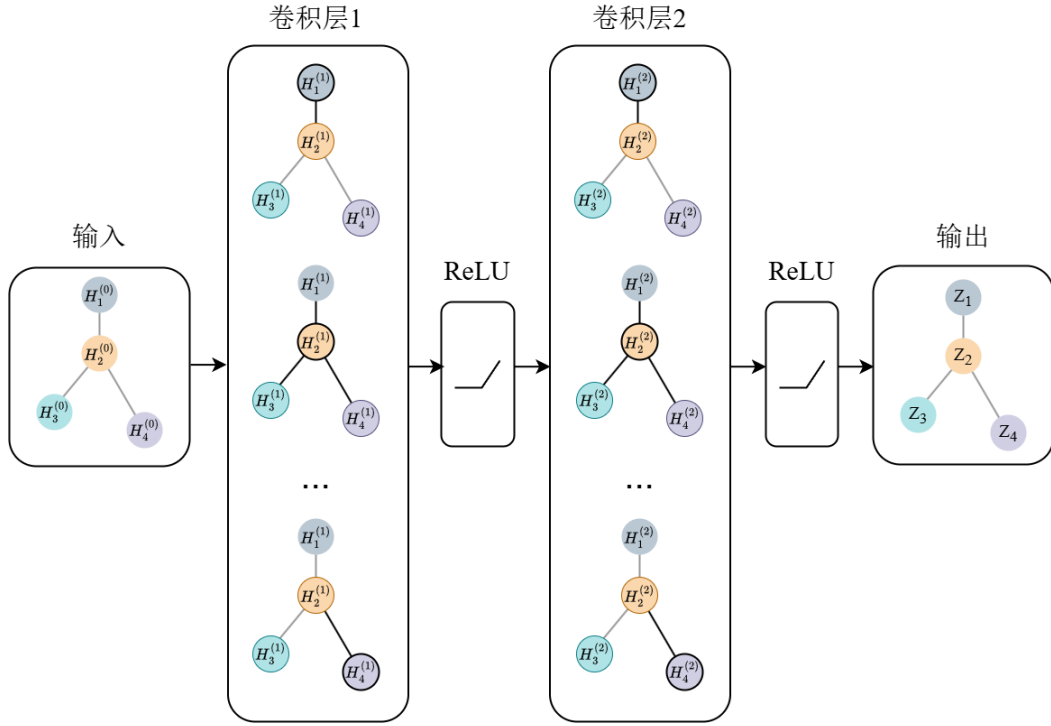
图 2-3 图卷积神经网络结构示意图
