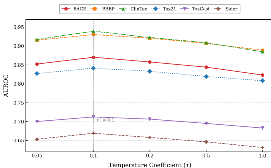
图 4-8 温度系数 \tau 对模型预测性能的影响
