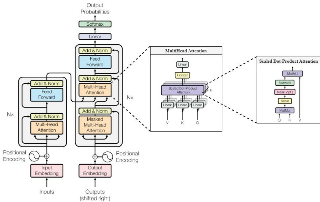
图 2-4 Transformer 架构
