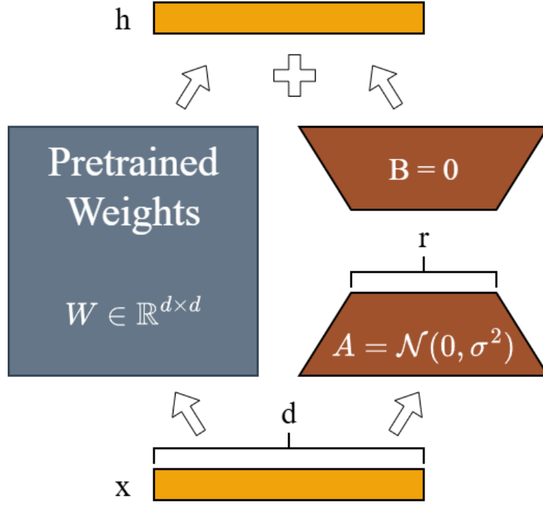
图 2-5 LoRA 技术原理示意图
