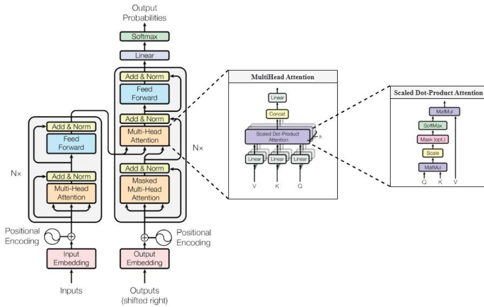
图 2-4 Transformer 架构 [50]
