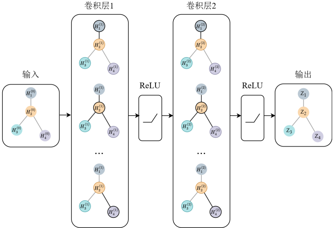
图 2-3 图卷积神经网络结构示意图
