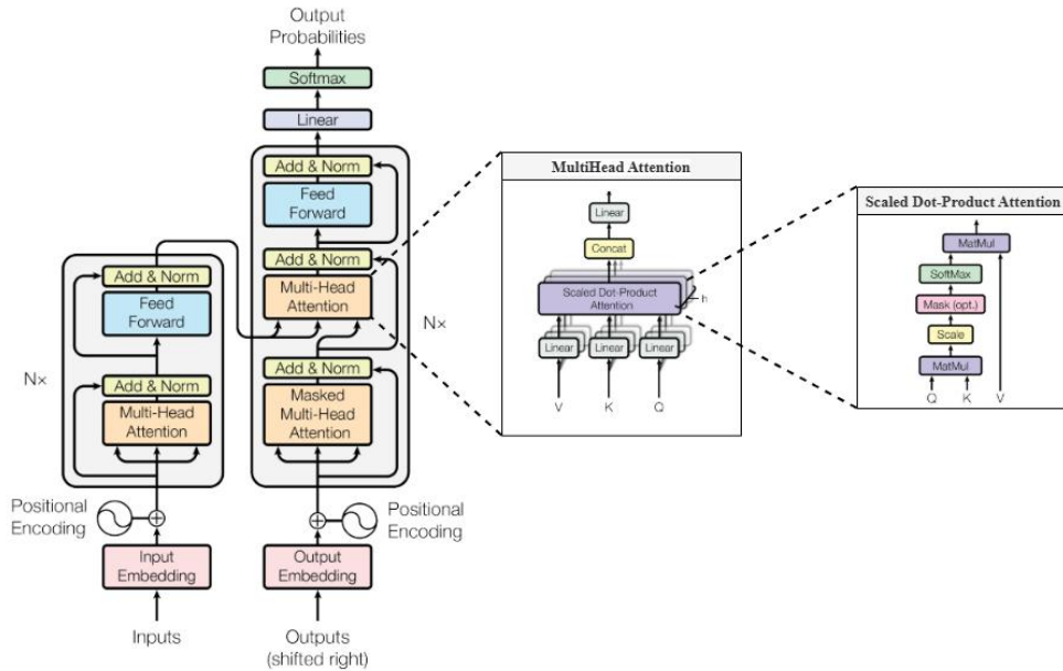
图 2-4 Transformer 架构 [51]
