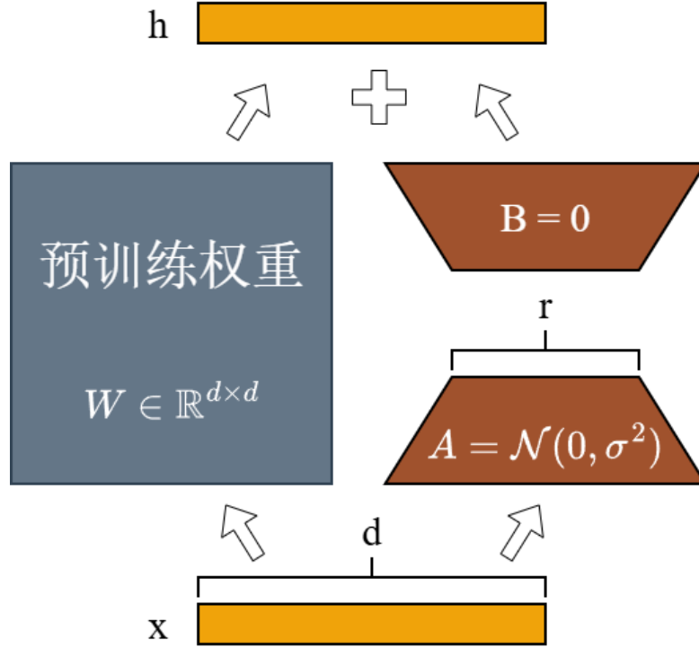
图 2-5 LoRA 技术原理示意图 [51]
