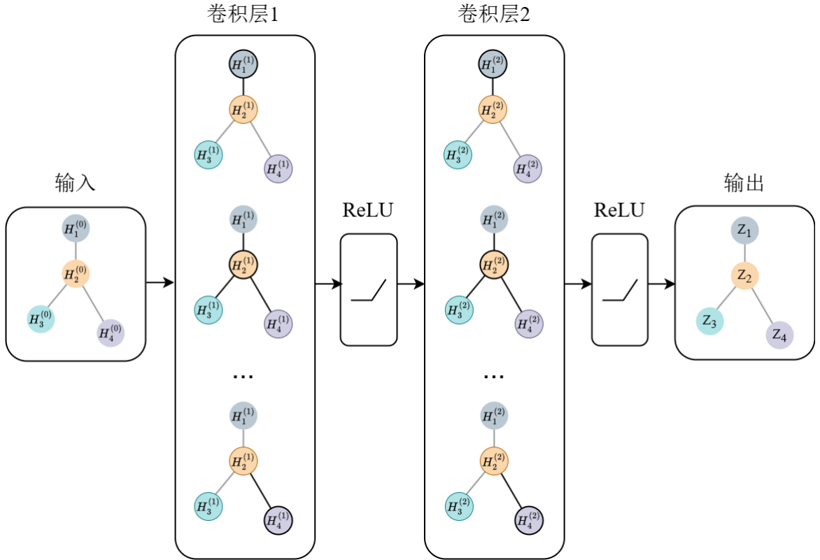
图 2-3 图卷积神经网络结构示意图
