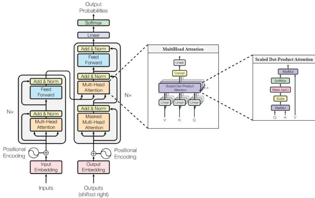
图 2-4 Transformer 架构 [49]
