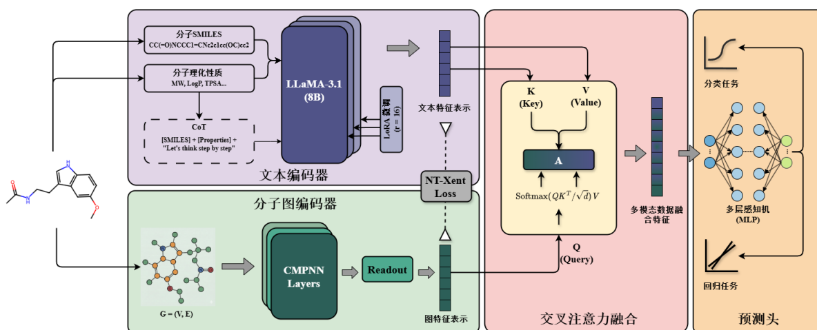
图 3-1 CoT-CMP 架构图
