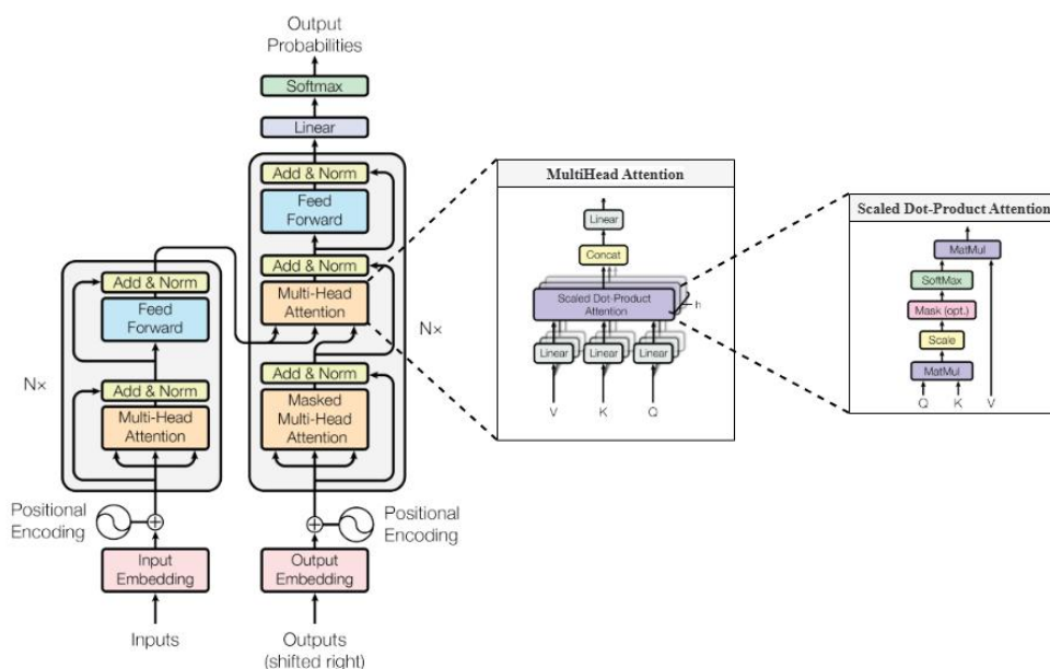
图 2-4 Transformer 架构
