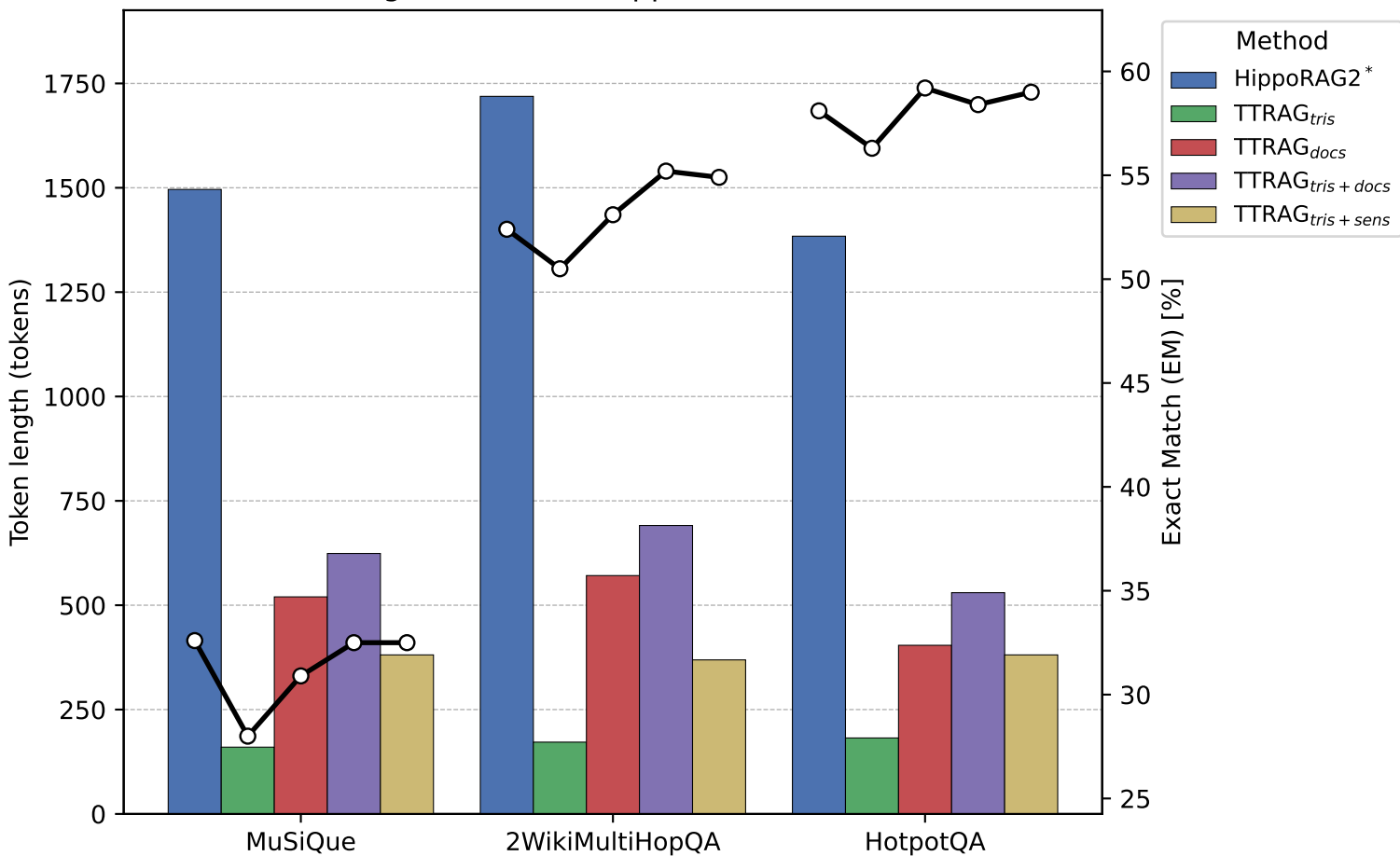
Token length and EM — HippoRAG2 (GPT-4o-mini)
