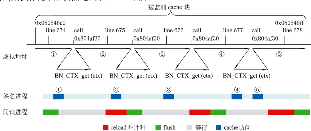
图 2 被监测 cache 块访问过程
