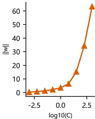
权重范数随正则化变化
