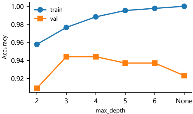
决策树深度与拟合程度
