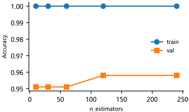
随机森林：树数 vs 性能
