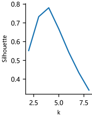
K 值与轮廓系数
