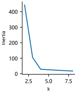
K 值与 SSE(Inertia)
