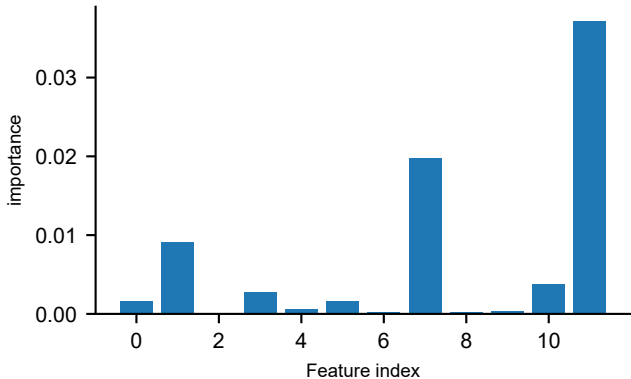
Fallback(GBDT) test acc=0.958
