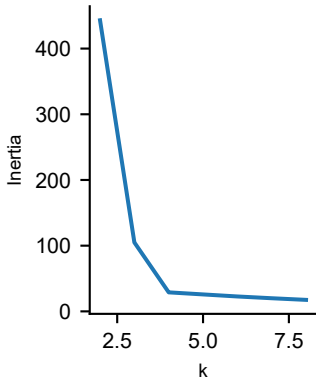
K 字 字 SSE(Inertia)
