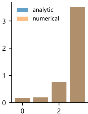
dW2: 解析 vs 数值
