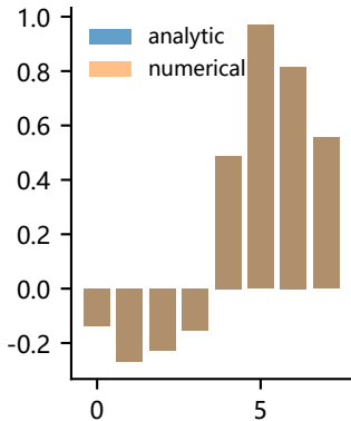
dW1: 解析 vs 数值
