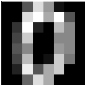
卷积核: blur
