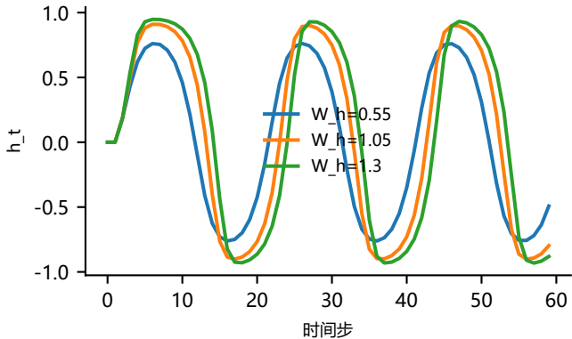
RNN 隐状态随时间演化
