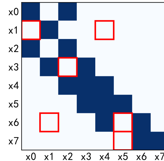
TS-GC (SNR=10dB)
