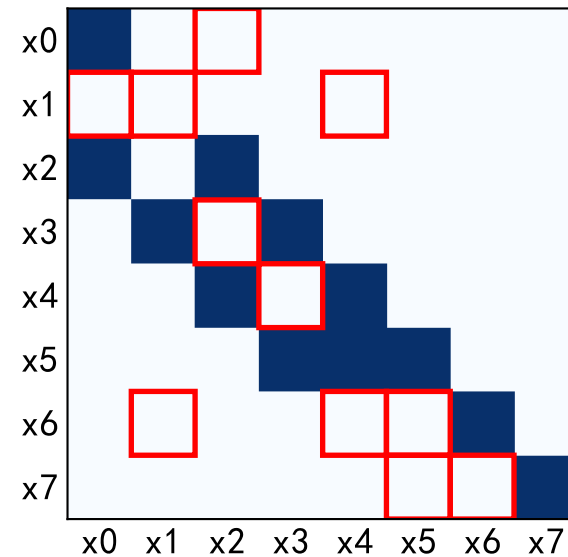
TS-GC (SNR=0dB)
