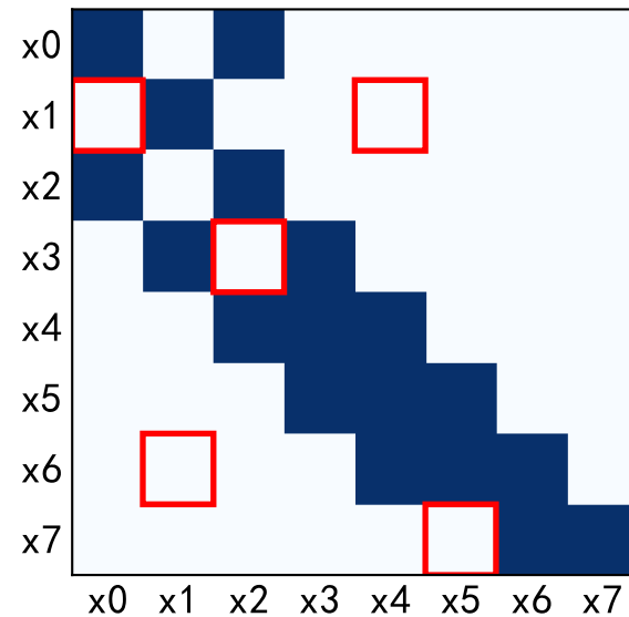
TS-GC (无SNR)
