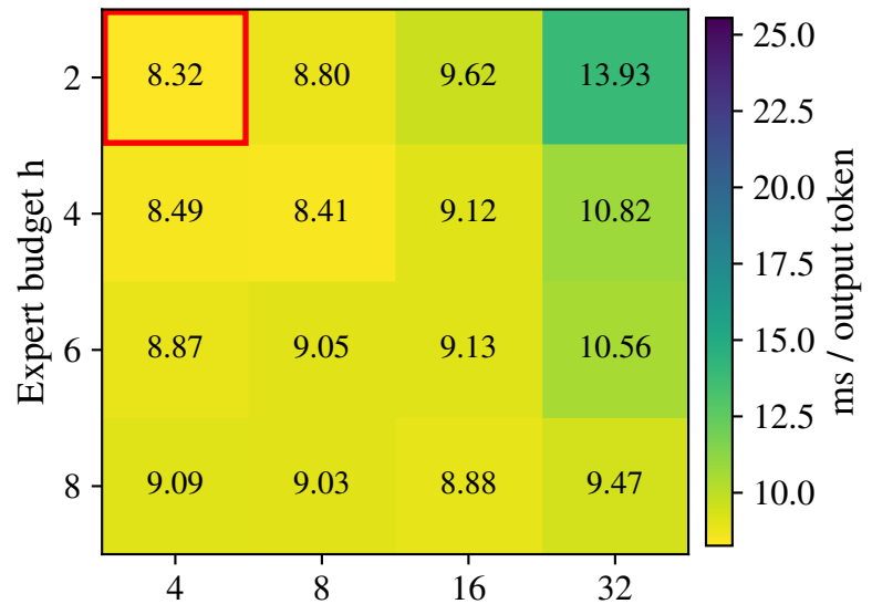
(d) Gemma4
