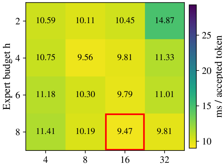
(c) Gemma4
