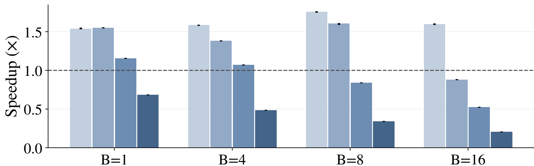
(b) E2E: baseline SD / AR
