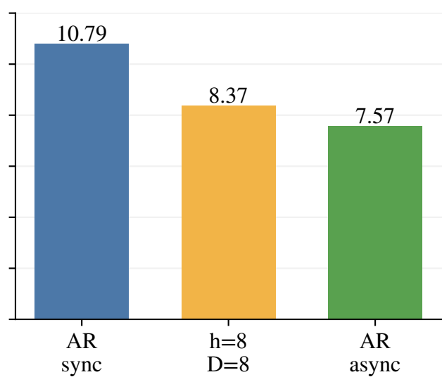
(b) Gemma4
