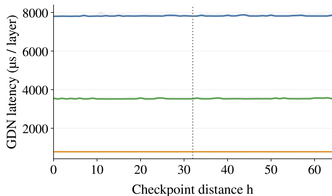
(d) Draft = 32
